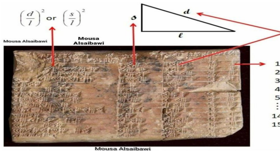
Plimpton 322 La tabla trigonométrica más antigua y precisa del mundo
